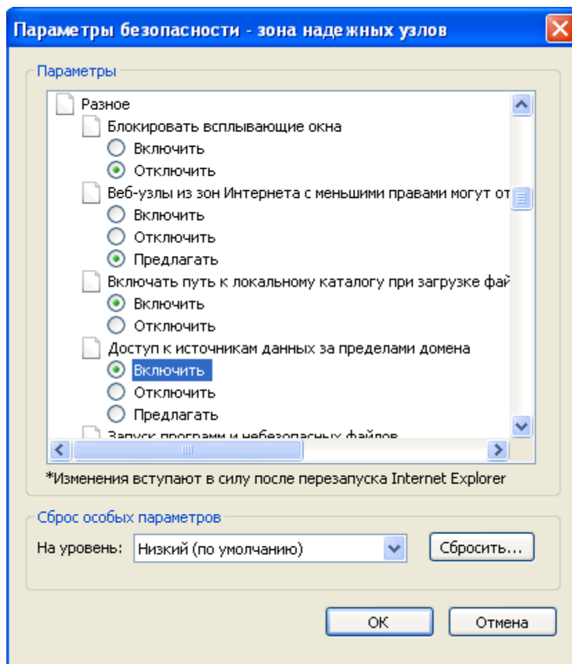
Рисунок 11. Настройка доступа
