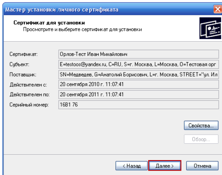
Рисунок 40. Данные сертификата
