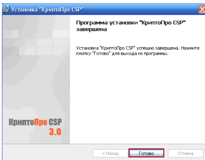
Рисунок 19. Окончание установки
