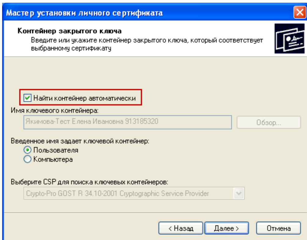
Рисунок 41. Определение контейнера
