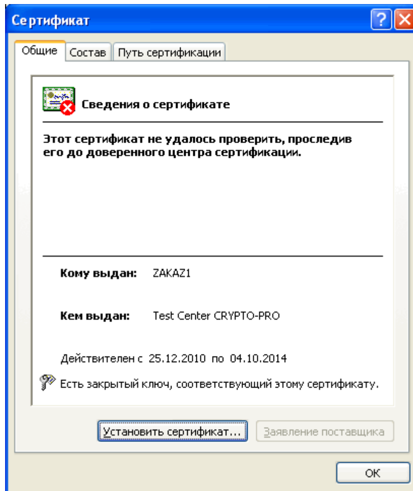
Рисунок 3. Сведения сертификата
