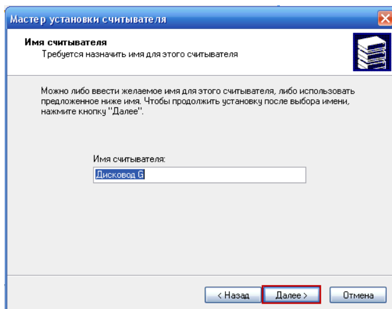
Рисунок 36. Имя считывателя
