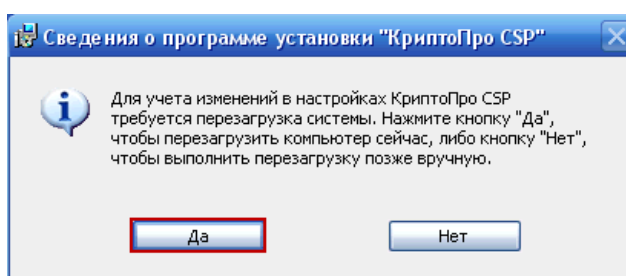
Рисунок 20. Перезагрузка
