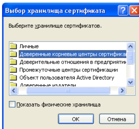
Рисунок 5. Список хранилищ
