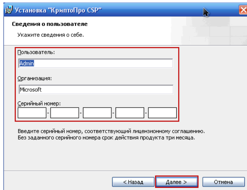
Рисунок 16. Серийный номер
