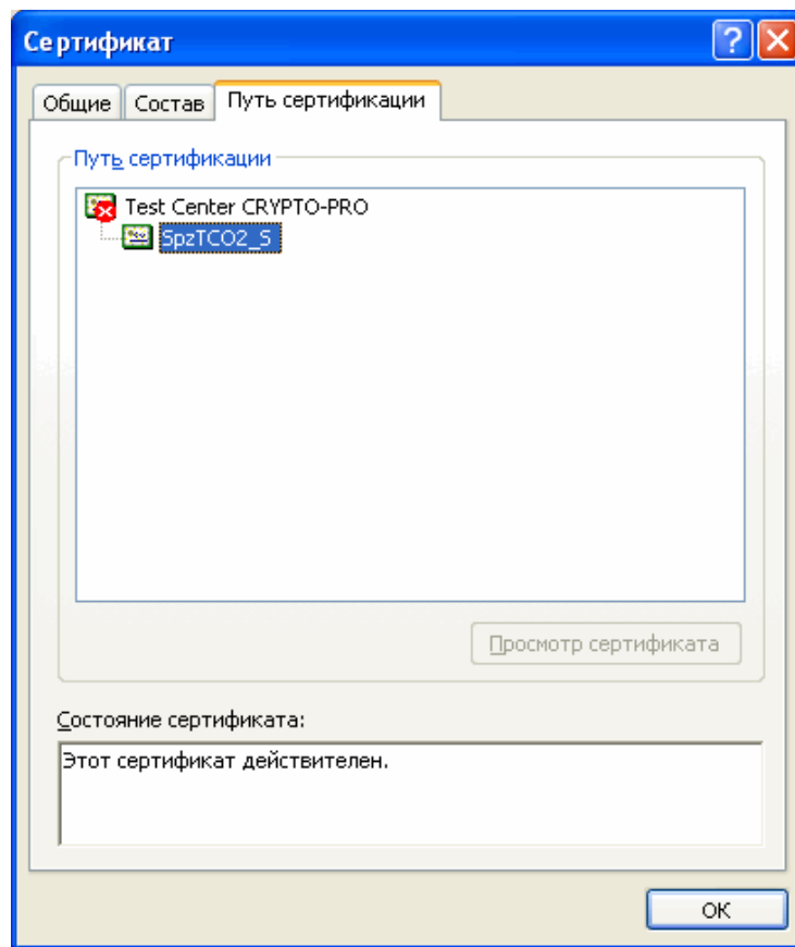
Рисунок 24. Сертификат
