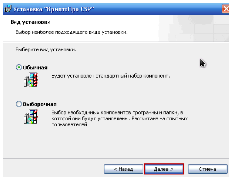
Рисунок 17. Вид установки
