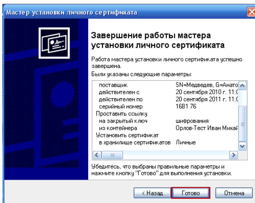
Рисунок 43. Окончание установки
