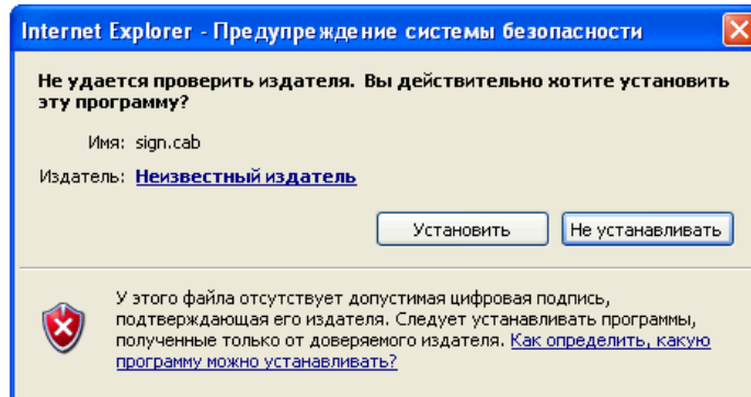
Рисунок 30. Установка компонента
