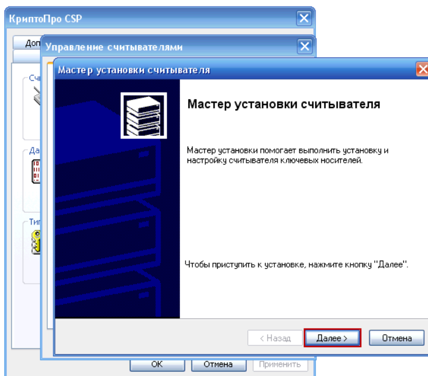
Рисунок 34. Установка считывателя
