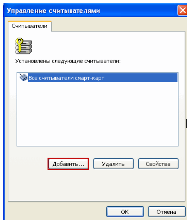
Рисунок 33. Добавление считывателя
