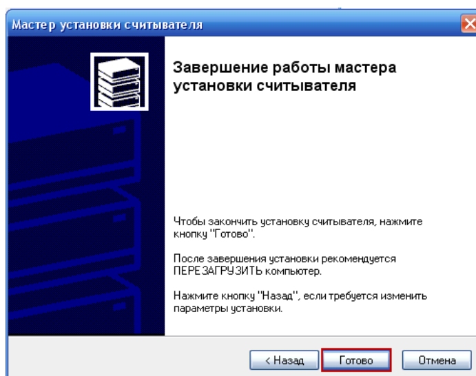
Рисунок 37. Окончание установки
