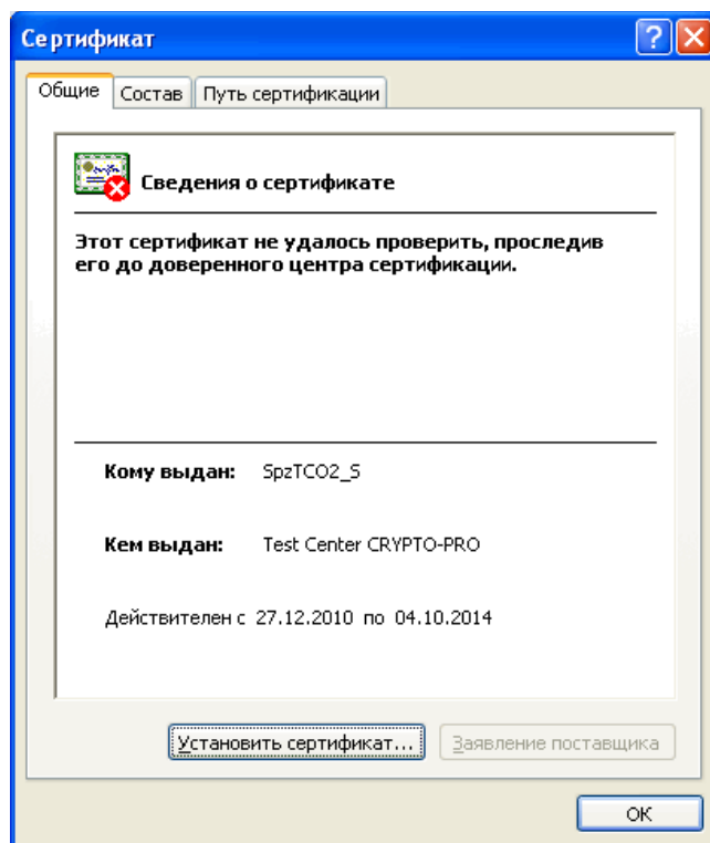
Рисунок 25. Корневой сертификат
