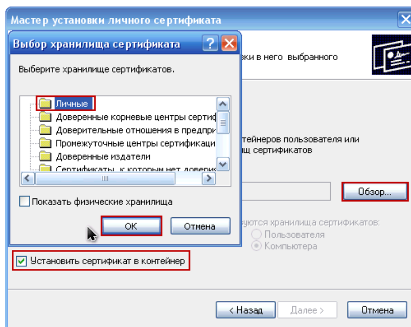
Рисунок 42. Выбор хранилища
