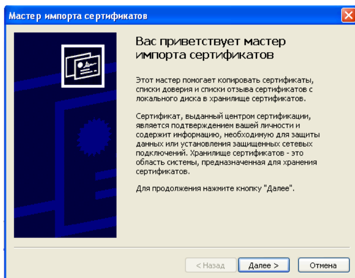
Рисунок 26. Импорт сертификата
