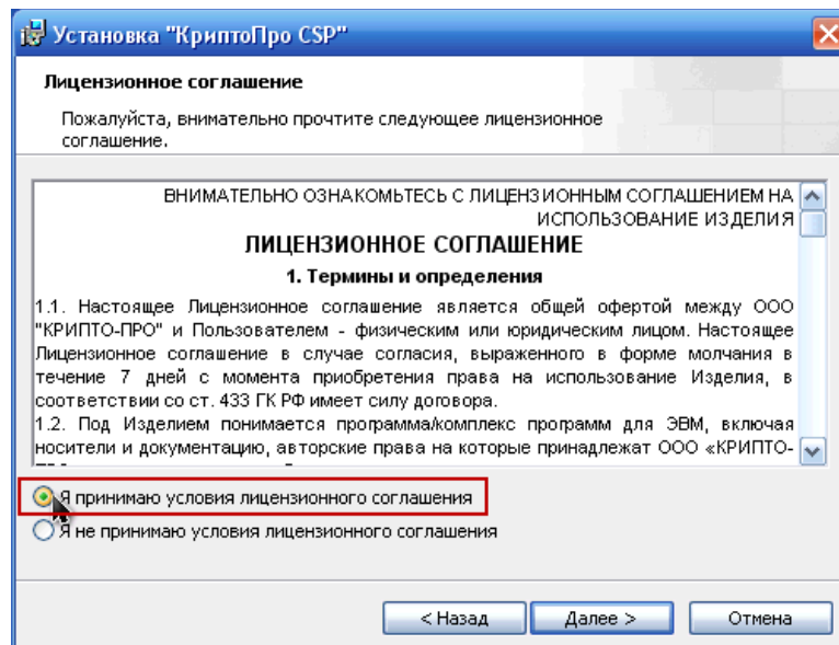
Рисунок 15. Лицензионное соглашение
