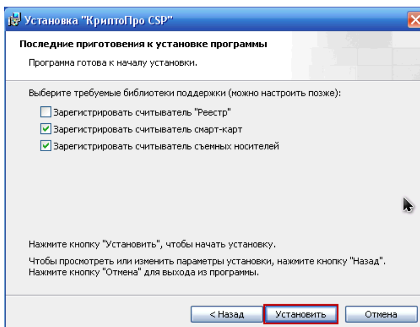
Рисунок 18. Типы считывателей
