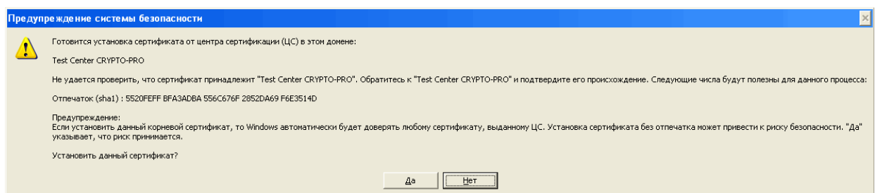
Рисунок 29. Подтверждение импорта
