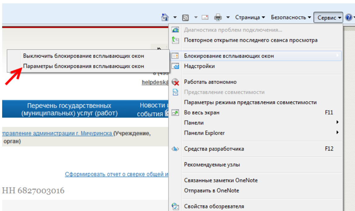
Рисунок 7. Всплывающее окно
